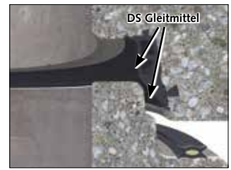
Beispiel: integrierte Schachtdichtung
