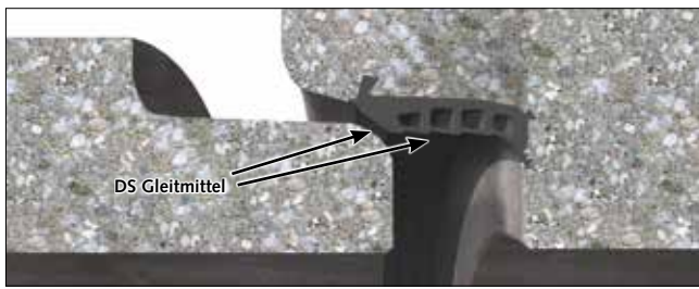
Beispiel: integrierte Rohrdichtung
